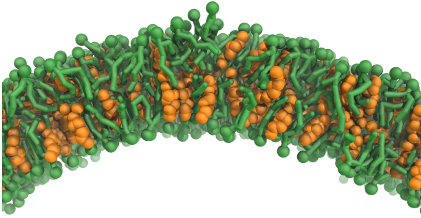
Abbildung 1: Die Abbildung zeigt ein Computermodell einer ungesättigten Membran. Diese besteht aus einer Lipid-Doppelschicht. Beim Verbiegen der Membran wandert das Cholesterin (orange) in die innere, negativ gekrümmte Lipidschicht. Diese Beweglichkeit von Cholesterin führt dazu, dass die Membran weicher wird, sich also leichter verbiegen lässt.
