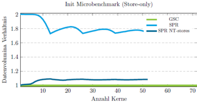
Abbildung 1: Store-only Benchmark auf je einem Sockel von GSC (72 Kerne) und SPR (52 Kerne). Die Y-Achse zeigt das Verhältnis von gemessenem Datentransfer vs. erwartetem Datentransfer (d.h. nur Speicherdatenvolumen).
